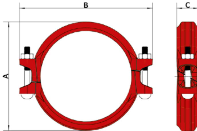
Ryc. 3. Konstrukcja złącza sztywnego typu XGQT1.
