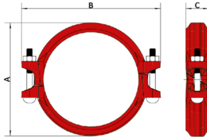
Ryc. 1. Wymiary złącza rurowego sztywnego rowkowego typu 1512.
