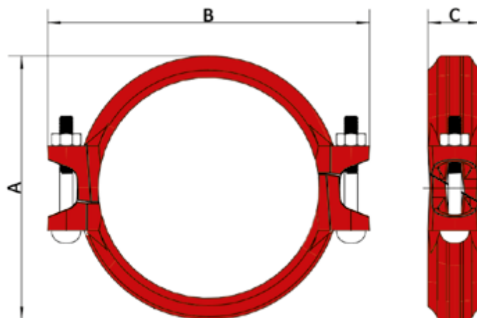
Ryc. 4. Konstrukcja złącza sztywnego typu XGQT4. Źródło: Materiały producenta.
