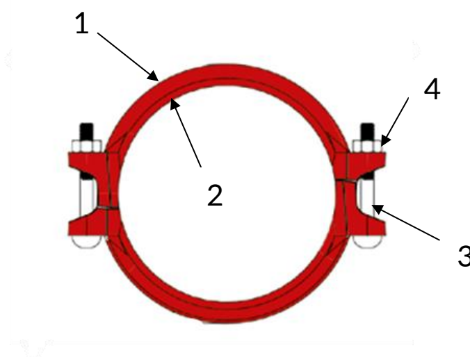
Ryc. 5. Konstrukcja złącza sztywnego (na przykładzie złącza typu XGQT4). 1- Korpus, 2- Uszczelka, 3- Śruba, 4- Nakrętka. Źródło: Materiały producenta.
