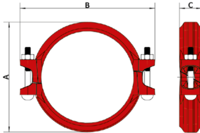
Ryc. 2. Wymiary złącza rurowego sztywnego rowkowego typu GKS. Źródło: Materiały producenta.
